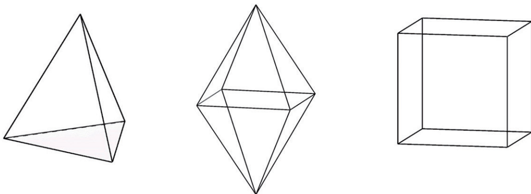
De Platonska kropparna tetraedern, oktaedern och hexaedern, det vill säga kuben.
